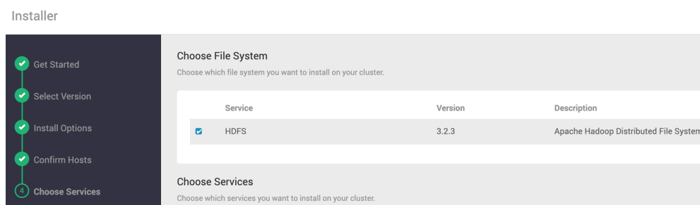
Figura 9 - Seleção do serviço da camada de armazenamento
