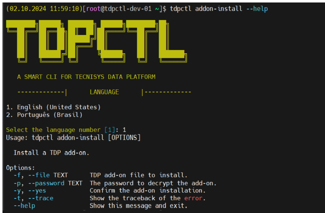
Figura 1 - Opção --help do comando tdpctl addon-install
