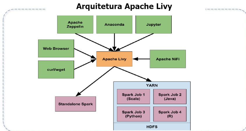
Arquitetura Apache Livy
