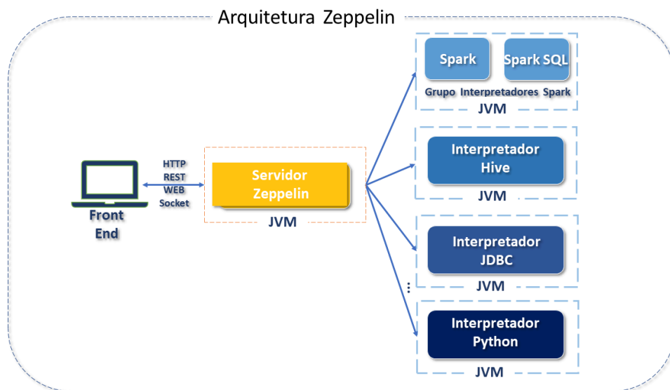
Arquitetura Zeppelin
