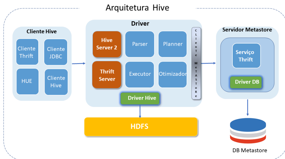
Figura 4 - Arquitetura Hive
