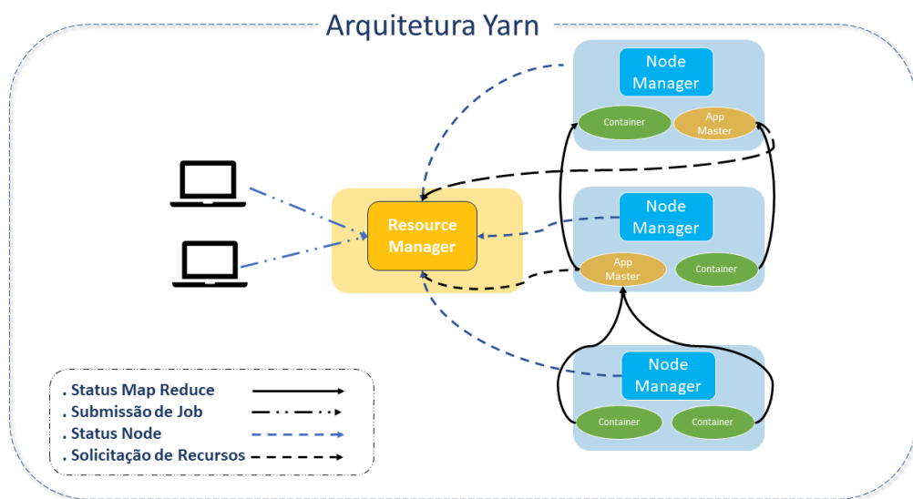
Arquitetura YARN
