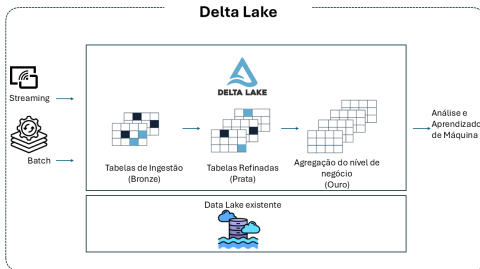
Figura 2 - Arquitetura do Delta Lake
