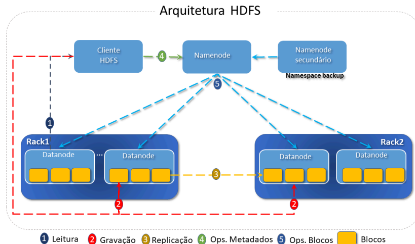
Figura 3 - Arquitetura HDFS
