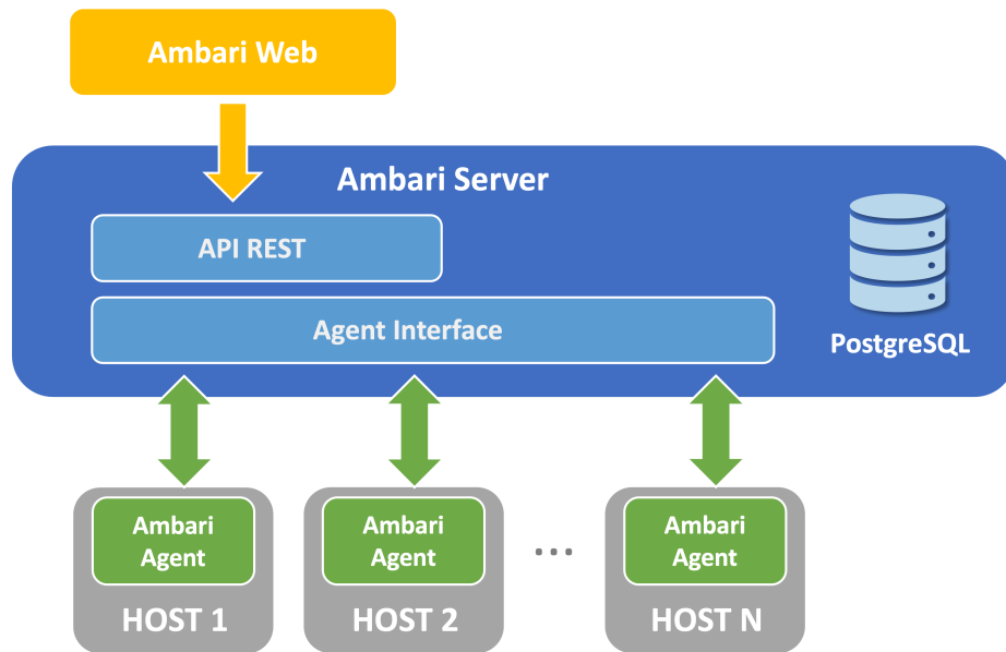
Figura 2 - Arquitetura do Ambari
