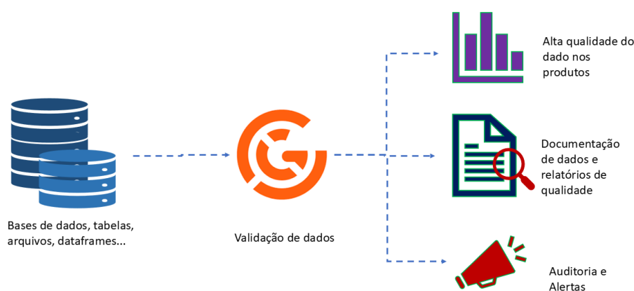
Figura 3 - Modelo do Great Expectations
