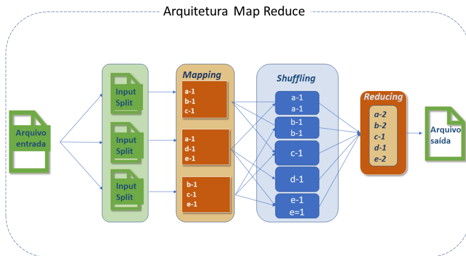
Arquitetura do Apache MapReduce
