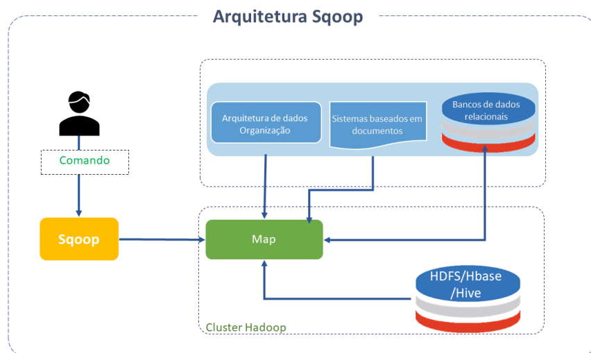
Arquitetura Sqoop
