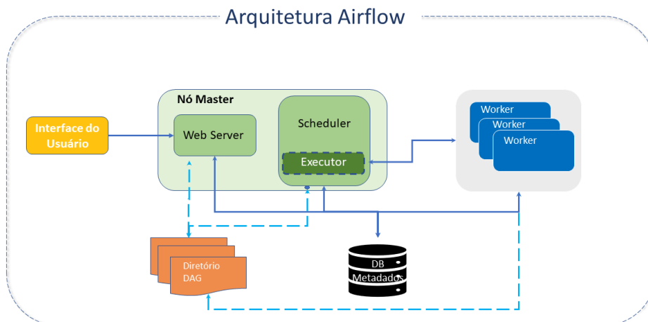
Figura 4 - Arquitetura Airflow
