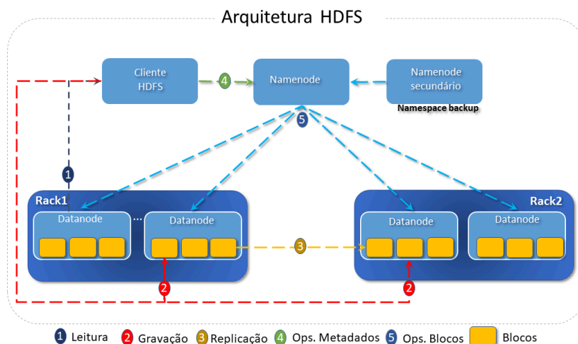
Figura 3 - Arquitetura HDFS
