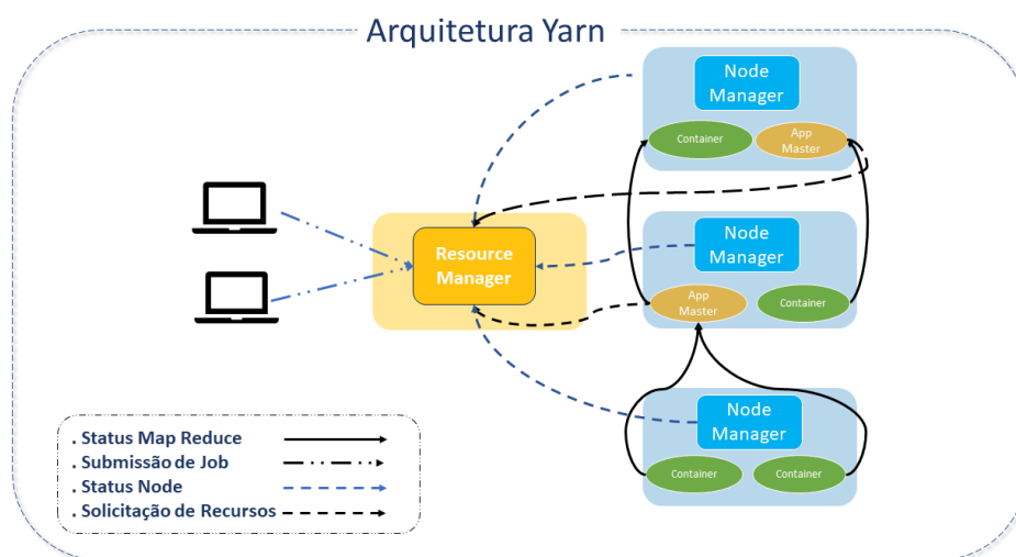
Arquitetura YARN
