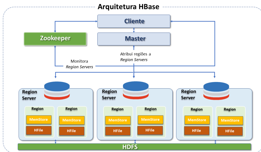
Figura 3 - Arquitetura HBase
