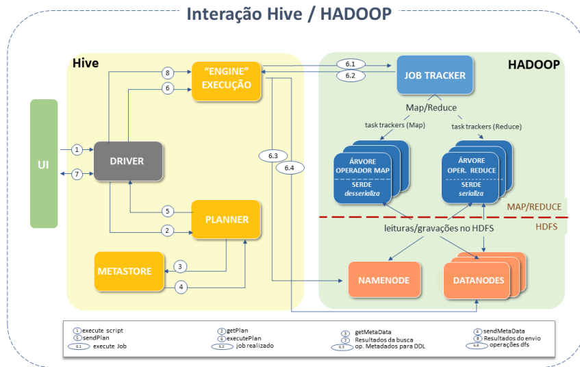
Figura 5 - Interação Hive-Hadoop
