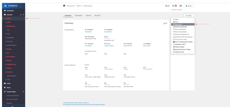
Figura 9 - Iniciar serviço
