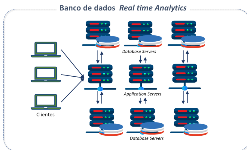
Computação Distribuída
