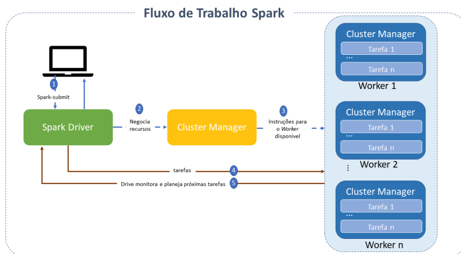
Fluxo Spark
