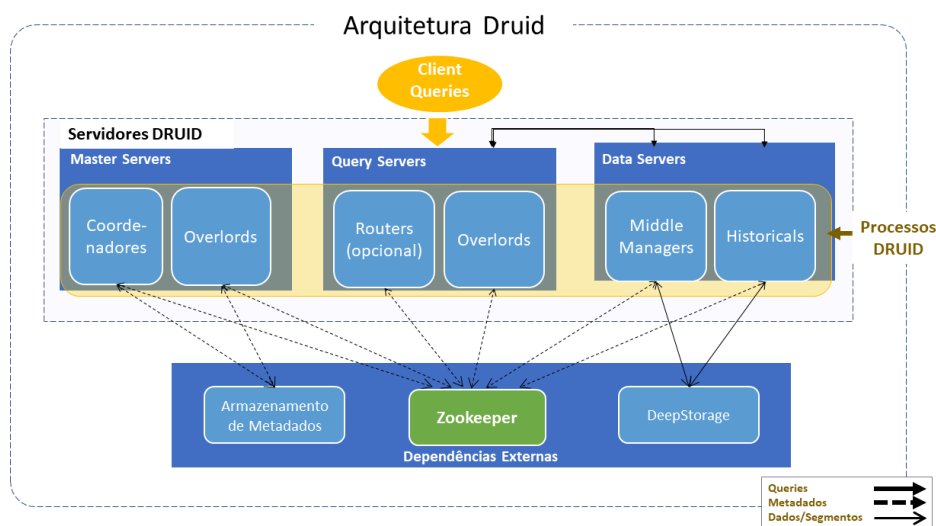
Figura 3 - Arquitetura Druid
