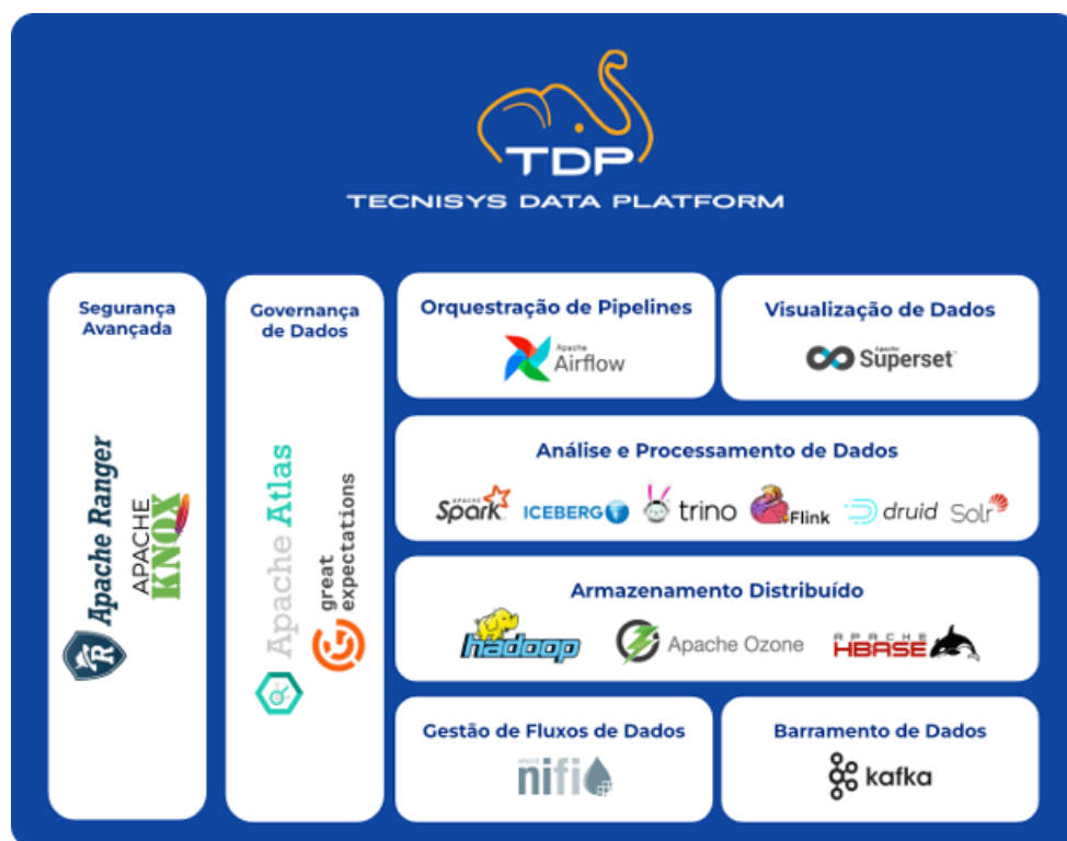
Figura 1 - Principais componentes
