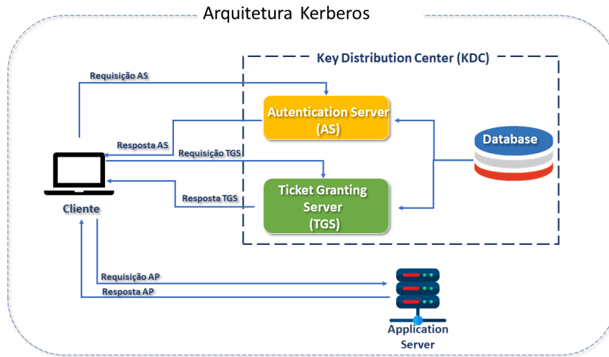
Arquitetura Kerberos
