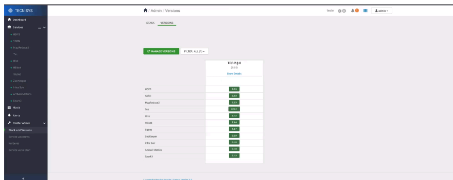
Figura 7 - Inconsistência resolvida
