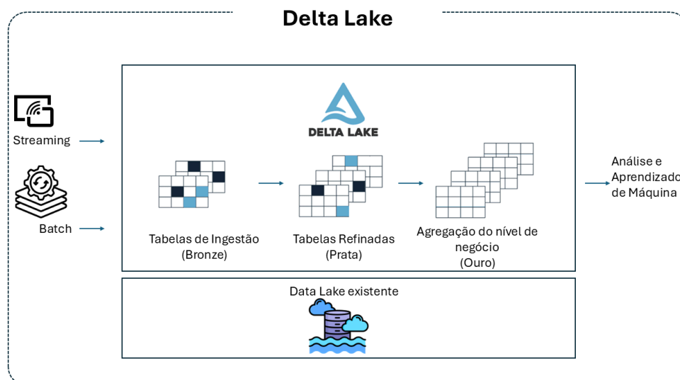
Figura 2 - Arquitetura do Delta Lake
