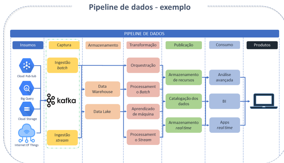
Figura 1 - Pipeline de dados
