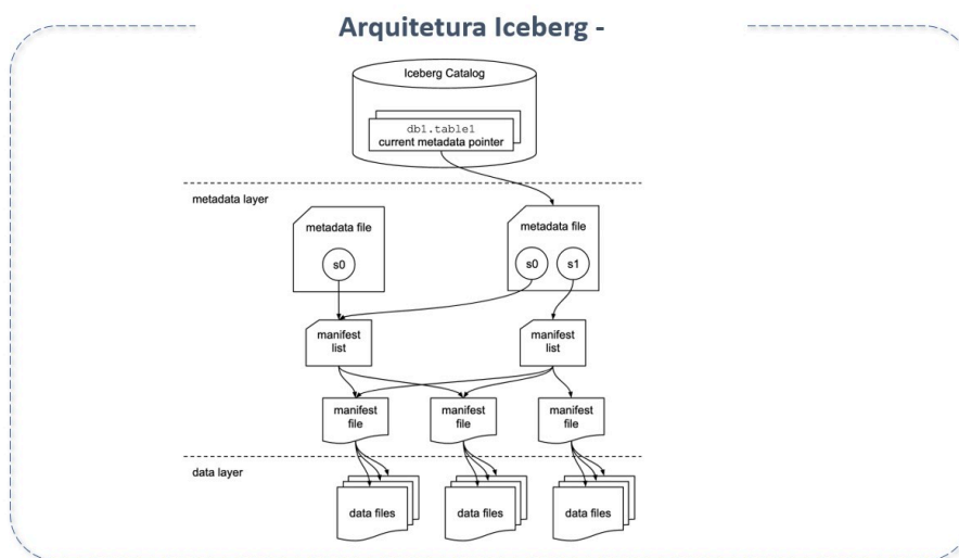
Arquitetura de uma tabela Iceberg
