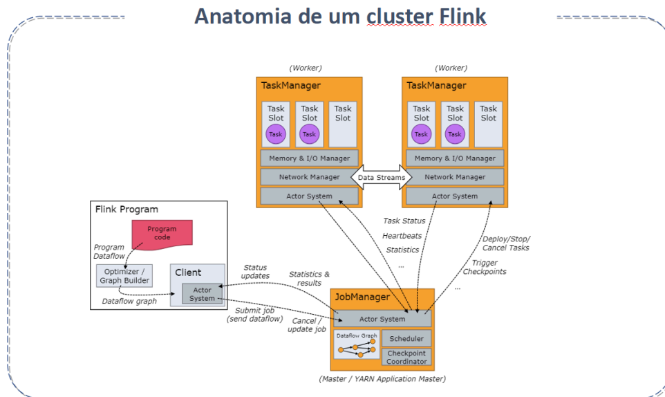
Figura 1 - Anatomia de um cluster Flink
