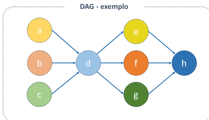
Figura 3 - Exemplo da estrutura de um DAG
