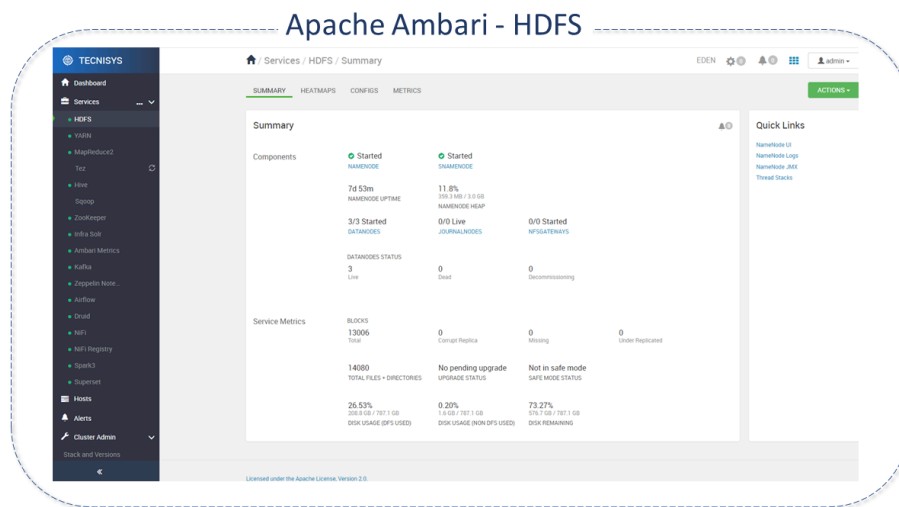
Figura 2 - Interface Ambari/HDFS
