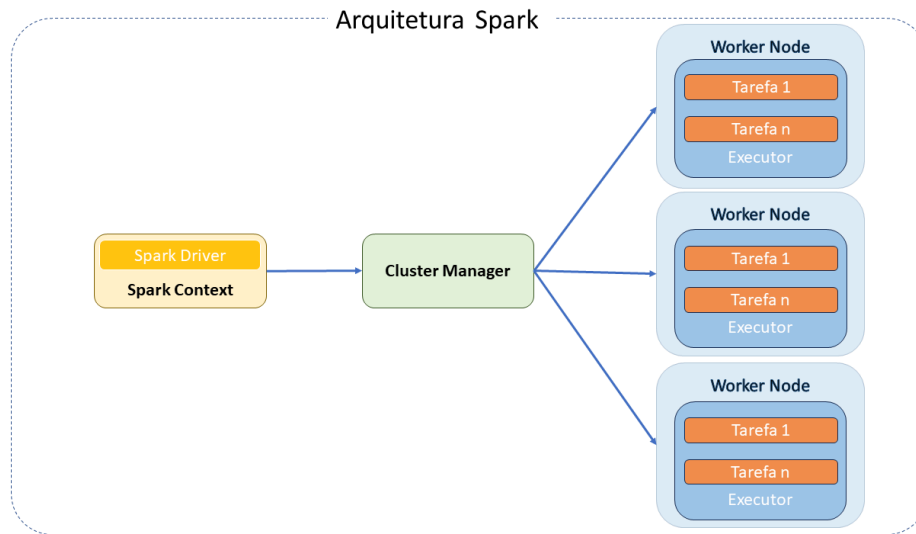
Arquitetura Spark
