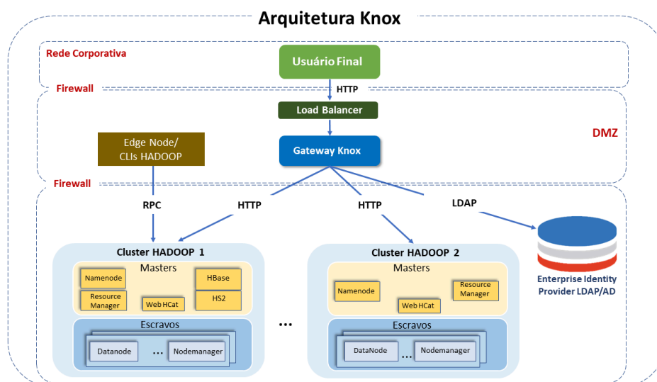
Arquitetura Knox
