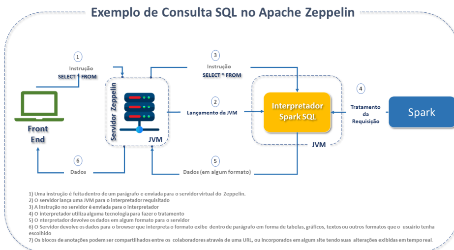
Exemplo Zeppelin
