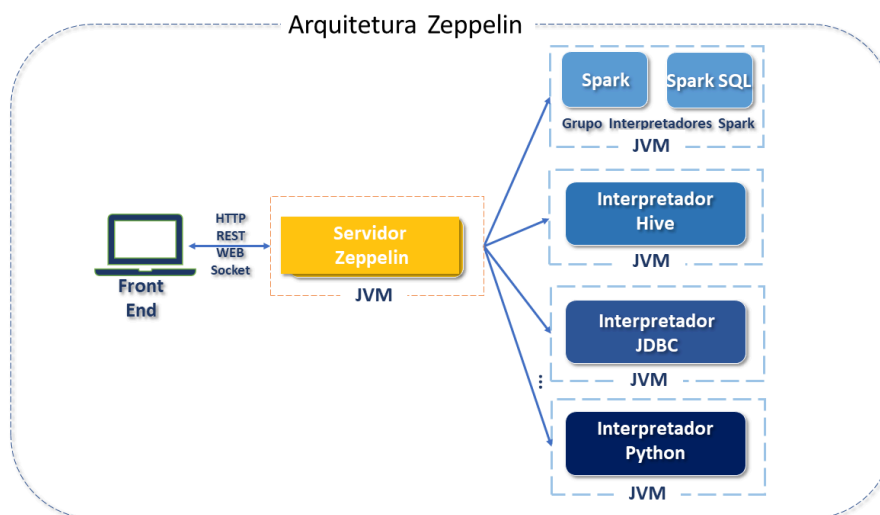
Arquitetura Zeppelin
