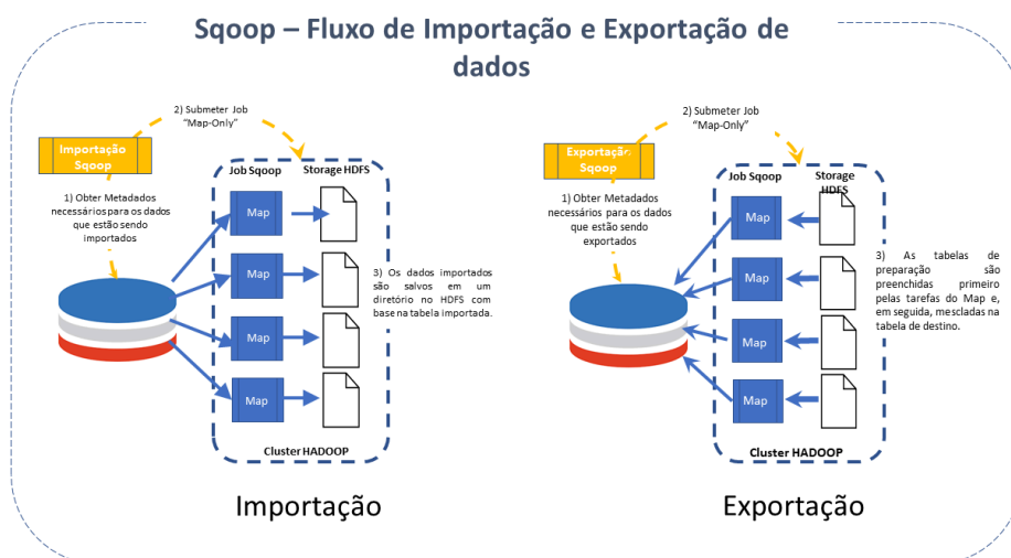
Fluxo Sqoop
