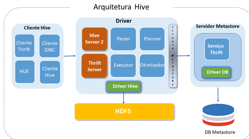
Figura 4 - Arquitetura Hive
