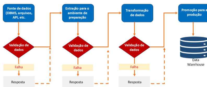
Figura 2 - Great Expectations - Validação de Dados
