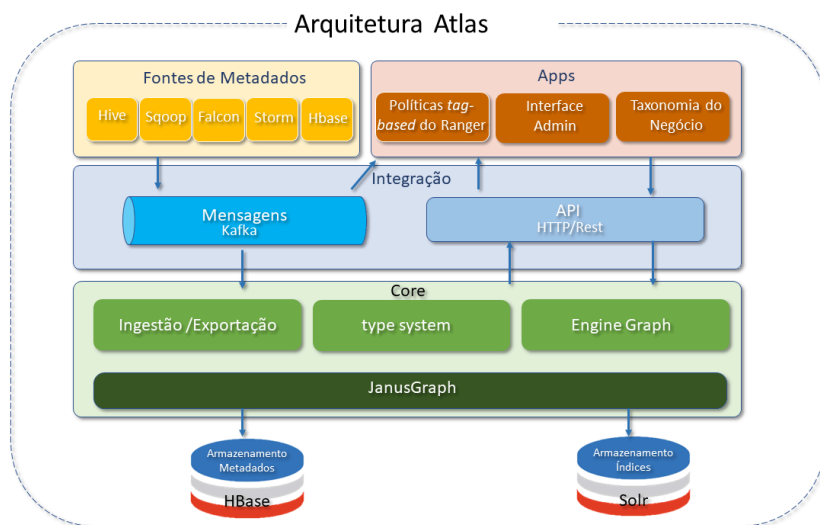
Figura 3 - Arquitetura Apache Atlas
